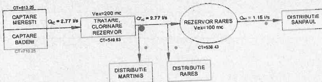
SCHEMA - SISTEM DE ALIMENTARE CU APA POTABILA MARTINIS
